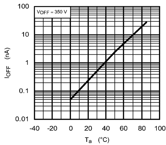
Fig. 14.9 I_{OFF} - T_a
