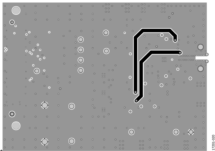
Figure 20. Layer 3
