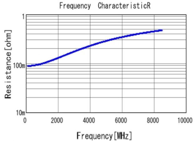
■ GCQ1555C1H6R5DB01 R DC0V, 25degC
