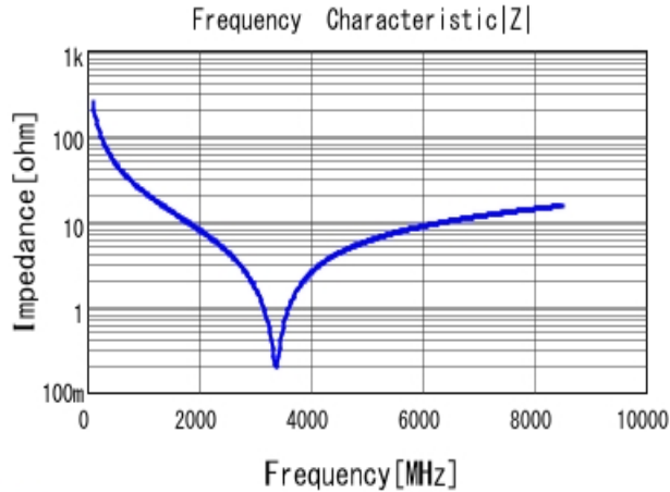
■ GCQ1555C1H6R5DB01 |Z| DC0V, 25degC
