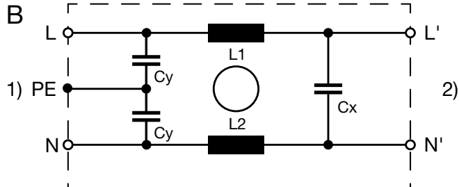
1) Line 2) Load
