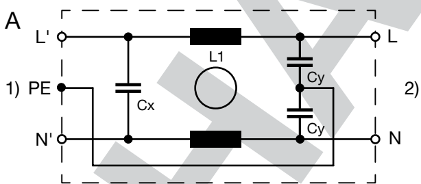
1) Line 2) Load
