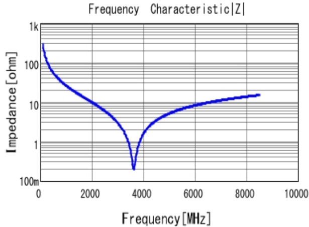
■ GCQ1555C1H5R6DB01 |Z| DC0V, 25degC
