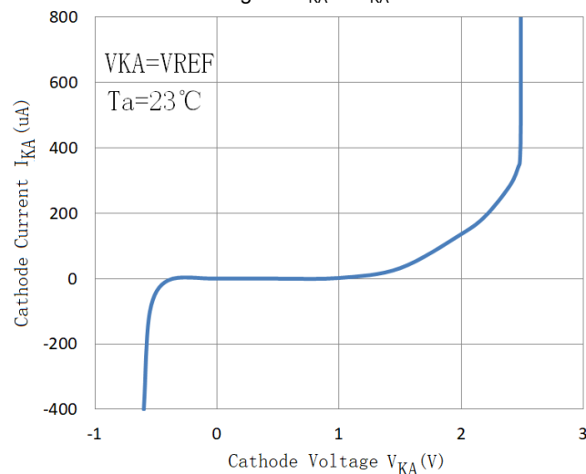
Fig. 2 - V_{KA} Vs I_{KA}
