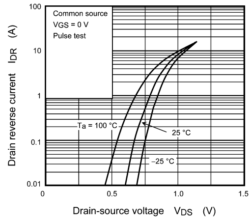
Fig. 9.8 I_{DR} - V_{DS}
