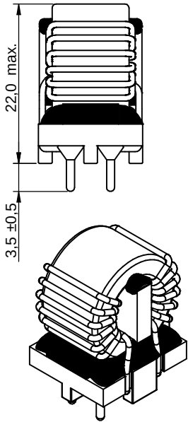
Scale - 1,5:1
