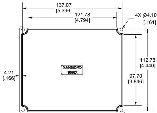
INSIDE LID
