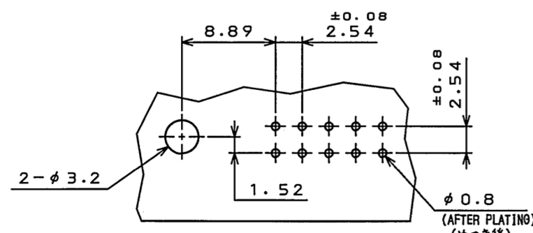
P.C.B. HOLE PATTERNS (REF.) 基板取付寸法(参考)
