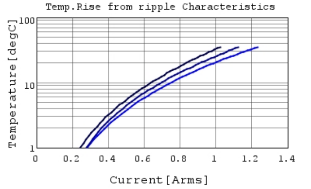
GRM1555C2A470JA01 Temp.rise 500MHz
