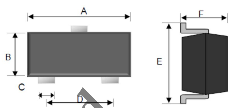
SOT-323
