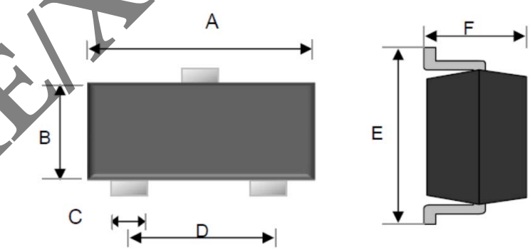
SOT-723
