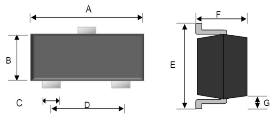
SOT-23
