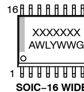
SOIC-16 WIDE
