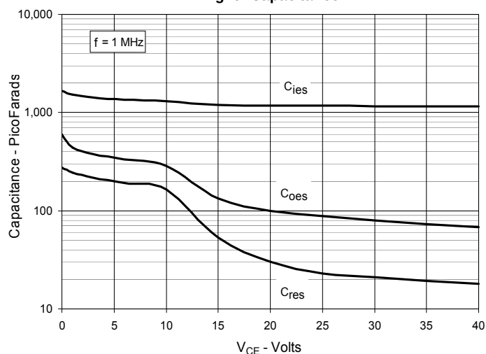
Fig. 9. Capacitance
