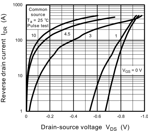
Fig. 8.6 I_{DR} - V_{DS}
