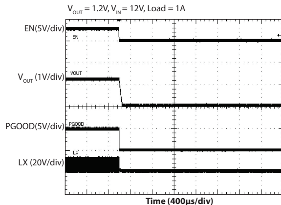
Shutdown via EN control
