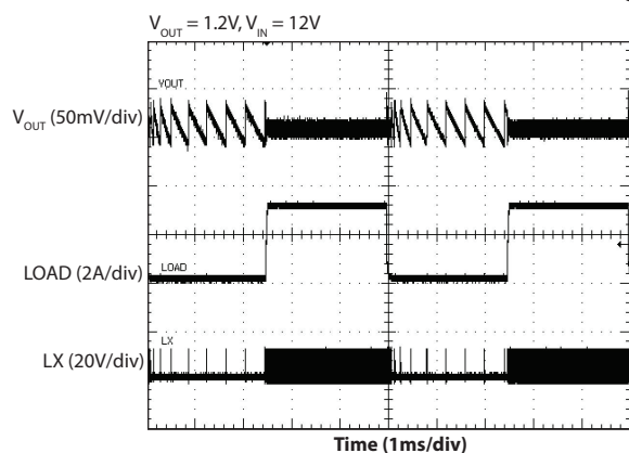
Load Transient, 0A to 3A to 0A - 1.5V OUT
