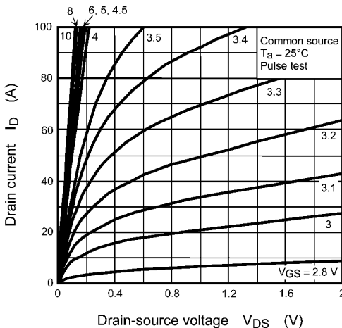
Fig. 8.2 I_D - V_{DS}
