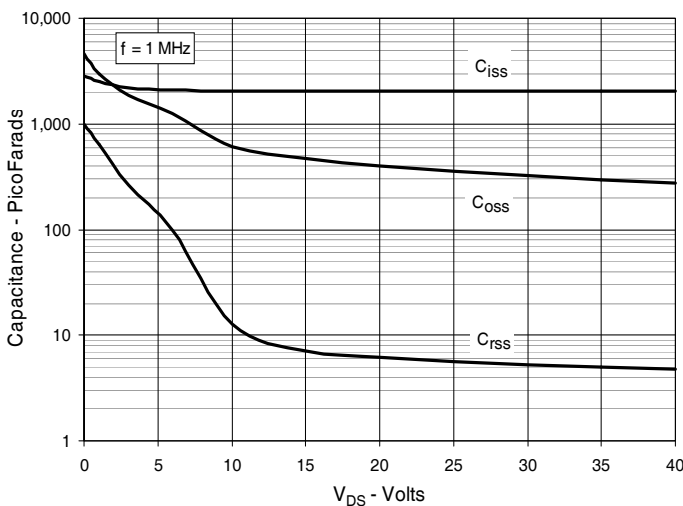
Fig. 11. Capacitance
