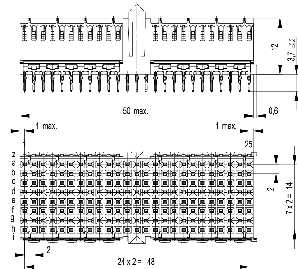
Bestückungsplan / contact layout
