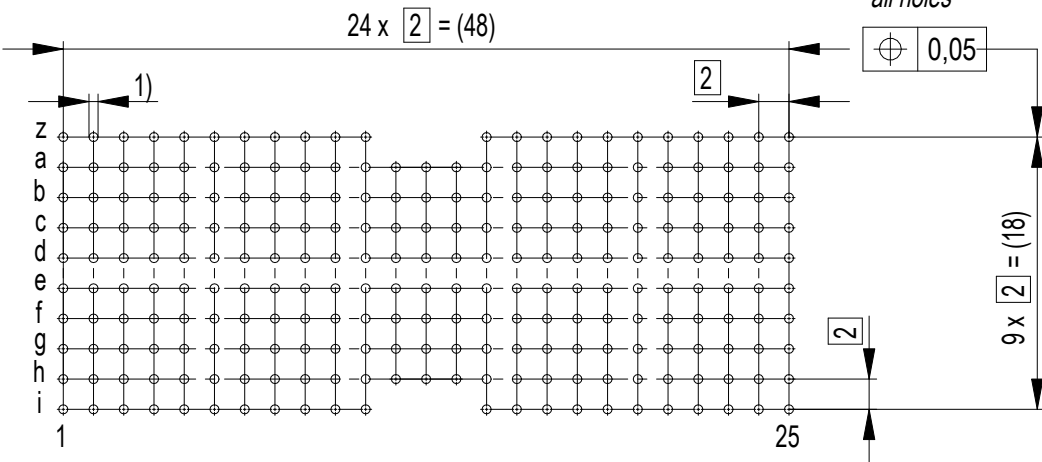
Lochbild für Leiterplatte (Bestückungsseite) board hole pattern (component mounting side)
