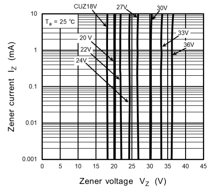
Fig. 10.1.2 I_Z - V_Z(2)
