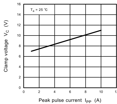
Fig. 10.4.2 V_C - I_{PP}
