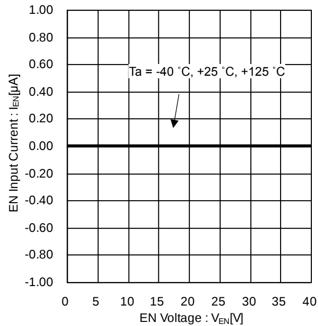
Figure 10. EN Input Current vs EN Voltage
