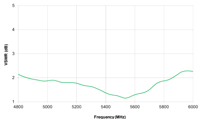
5 GHz VSWR
