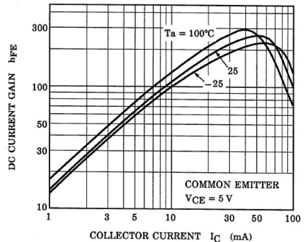
Fig. 10.14 RN1902 h_{FE} - I_C
