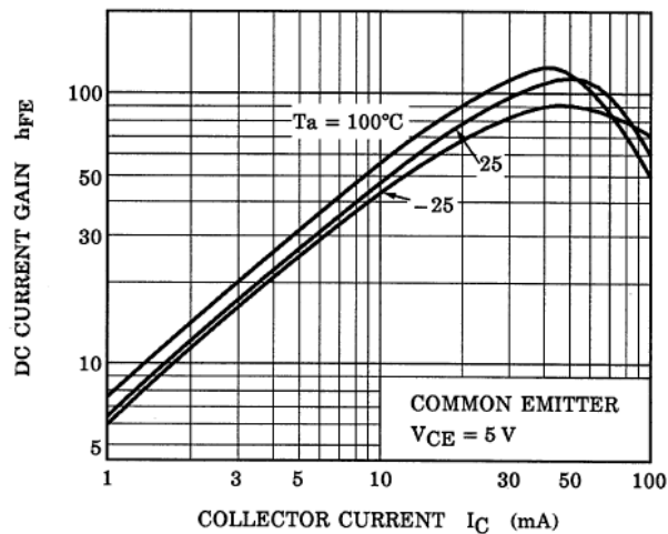
Fig. 10.13 RN1901 h_{FE} - I_C
