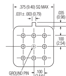
MGS/MGSD/MGSDD Header
