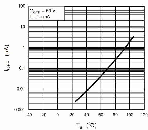
Fig. 12.8 I_{OFF} - T_a
