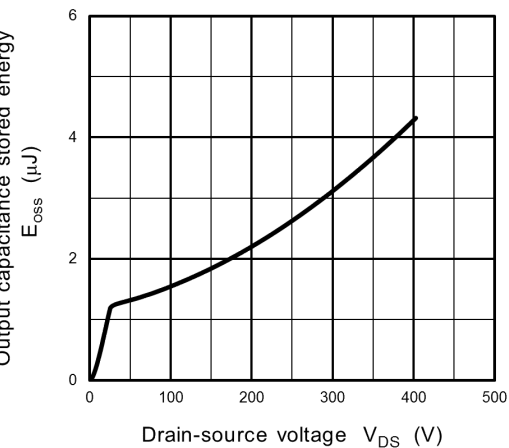
Fig. 8.12 E_{oss} - V_{DS}
