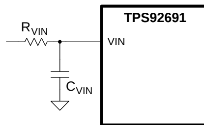
Figure 28. VIN Filter
