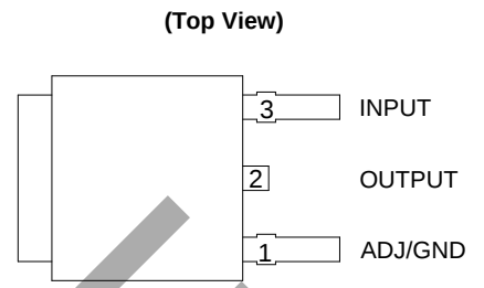
TO252-2 (5)
