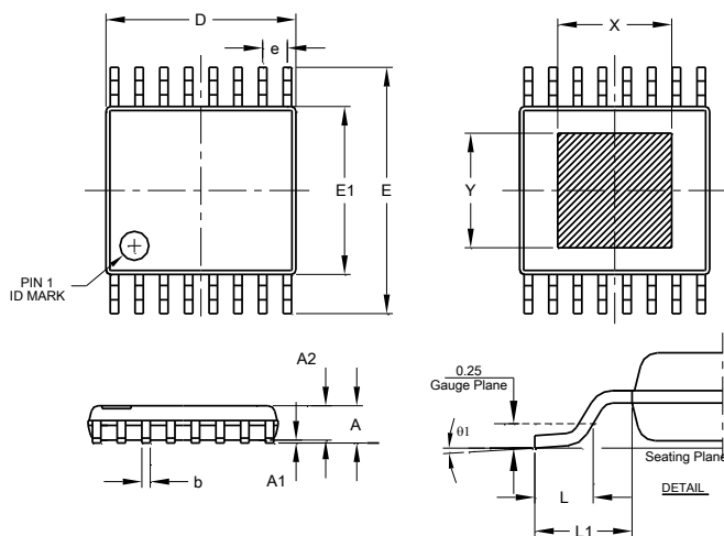
TSSOP-16EP
