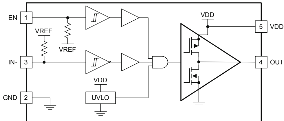
Figure 34. UCC27536
