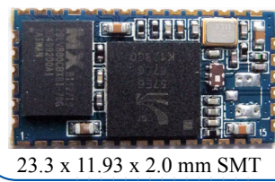
23.3 x 11.93 x 2.0 mm SMT
