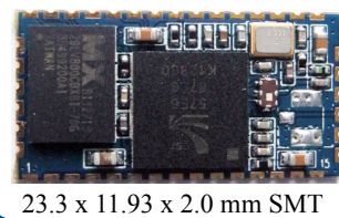
23.3 x 11.93 x 2.0 mm SMT
