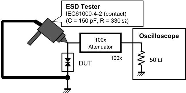
Fig. 5.1.3 IEC61000-4-2 (Contact)
