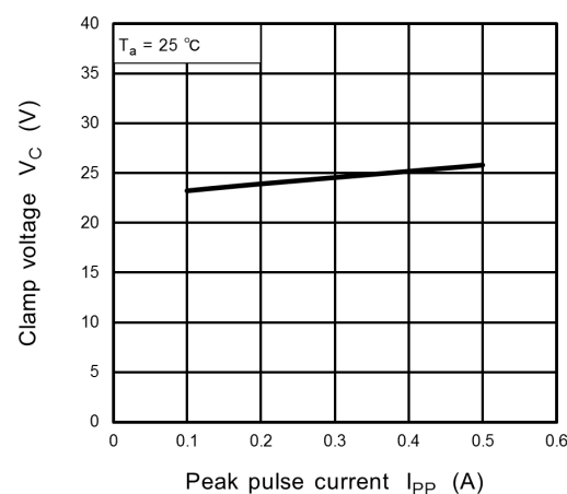
Fig. 5.3.1 V_C - I_{PP}
