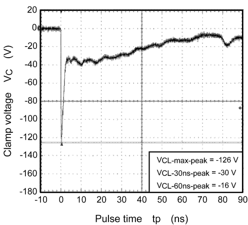
Fig. 5.1.2 -8 kV
