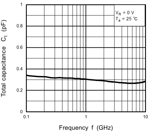
Fig. 8.4 C_t - f
