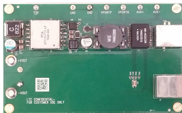
Bottom Side
