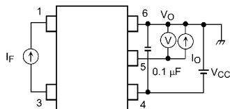
Fig. 12.1.3 V_{OH} Test Circuit
