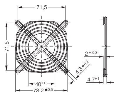
LZ32-4 Fan size 80 x 80
