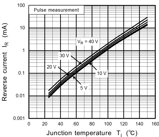
Fig. 10.8 I_R - T_j
