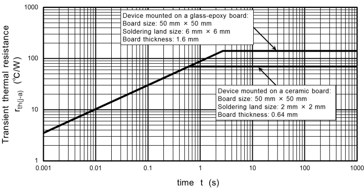
Fig. 10.6 r_{th(j-a)} - t
