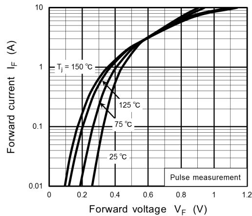
Fig. 10.1 I_F - V_F
