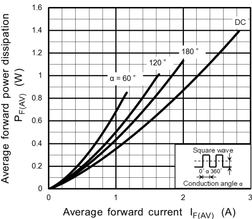
Fig. 10.2 P_{F(AV)} - I_{F(AV)}
