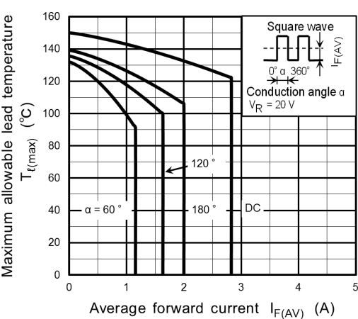
Fig. 10.4 T_{l(max)} - I_{F(AV)}
