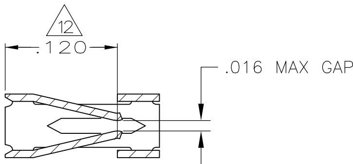
SECTION D-D
