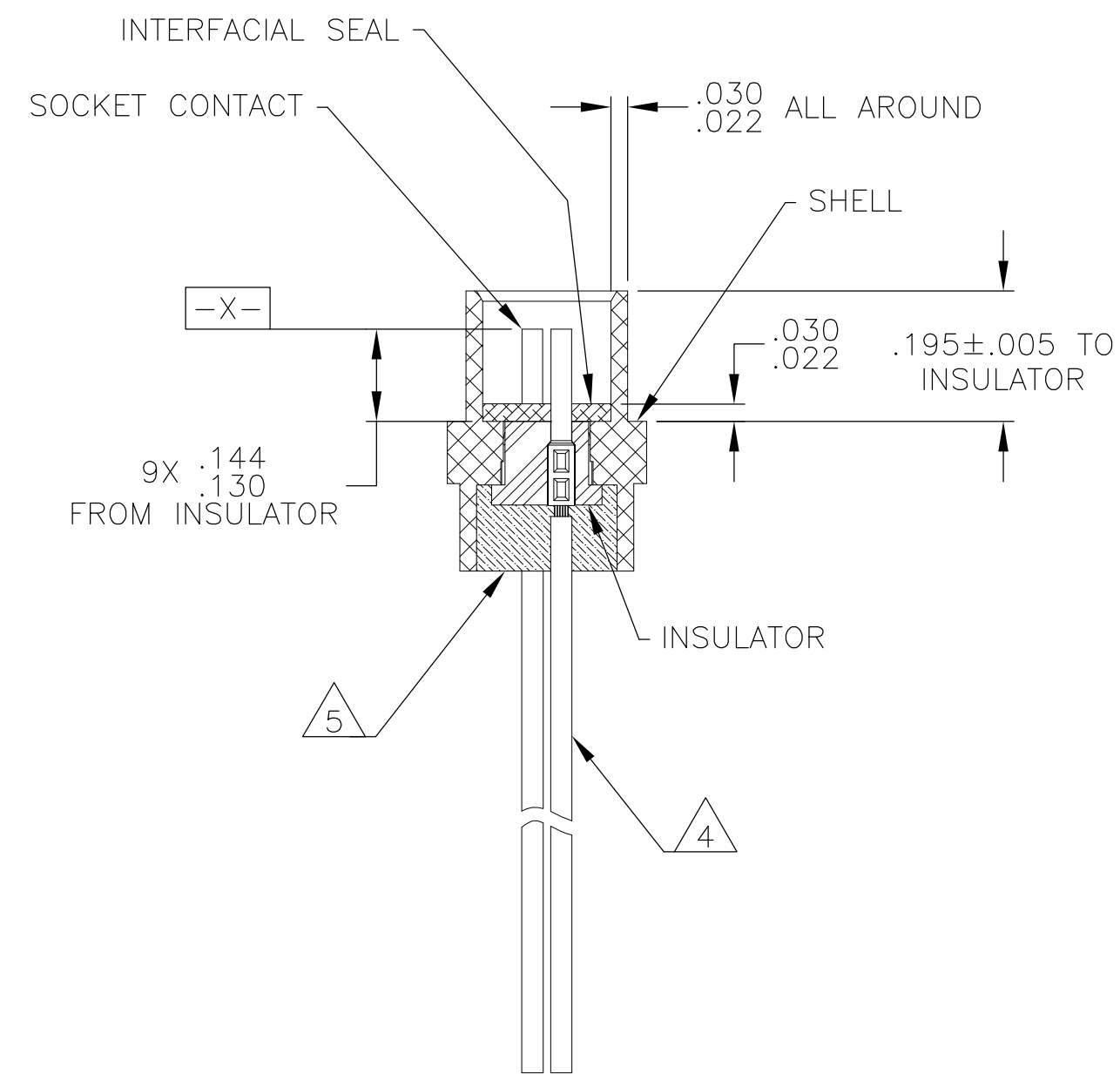
SECTION A-A
