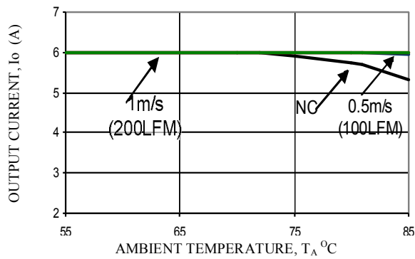
V_o=1.8V
