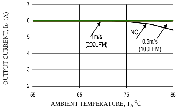
V_o=0.6V
