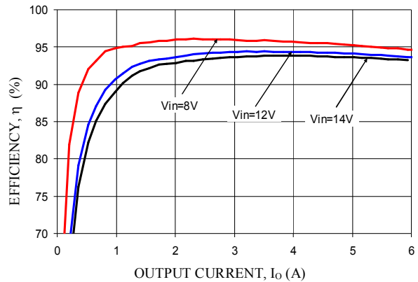
V_o = 5.0V
