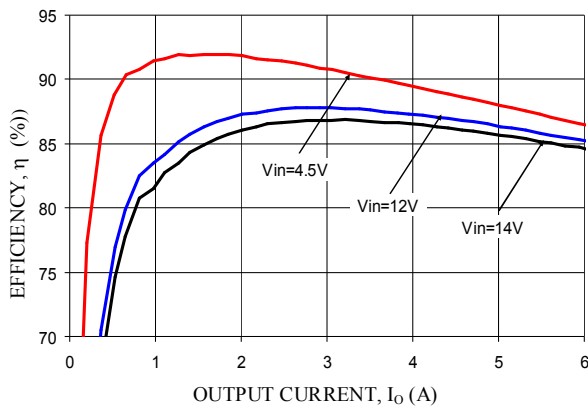
V_o = 1.8V
