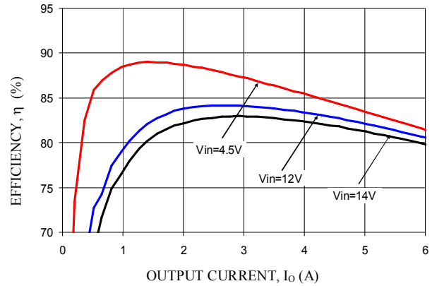
V_o = 1.2V
