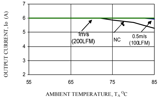
V_o=2.5V
