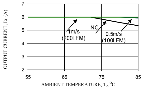
V_o=1.2V
