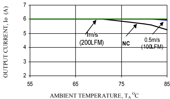
V_o=3.3V
