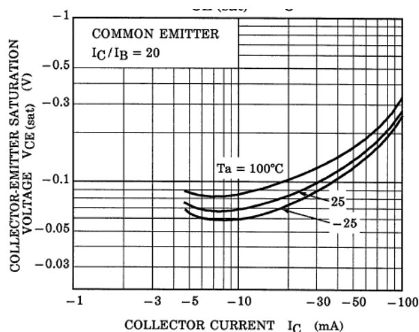
Fig. 10.19 RN2901FE V_{CE(sat)}-I_C
