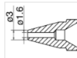
N61-10 Nozzle
