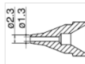
N61-06 Nozzle
