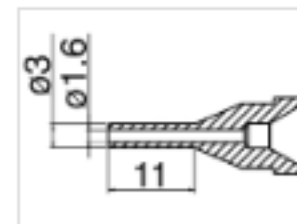
N61-14 Nozzle
