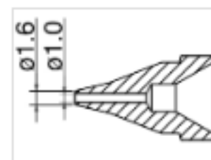
N61-03 Nozzle
