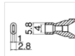
N61-16 Nozzle
