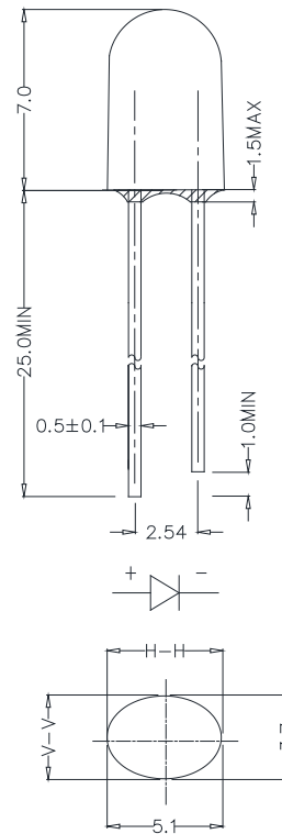
C5SMF-RJE/GJE/BJE:
