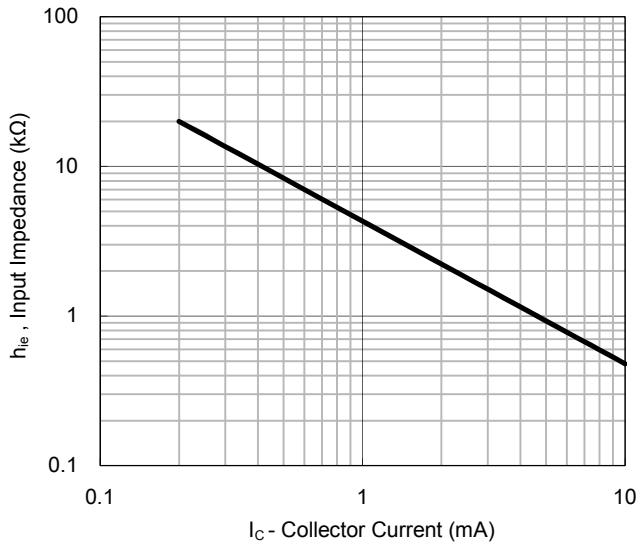
Fig.9 Input Impedance
