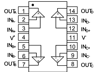
SOP-14L / TSSOP-14L
