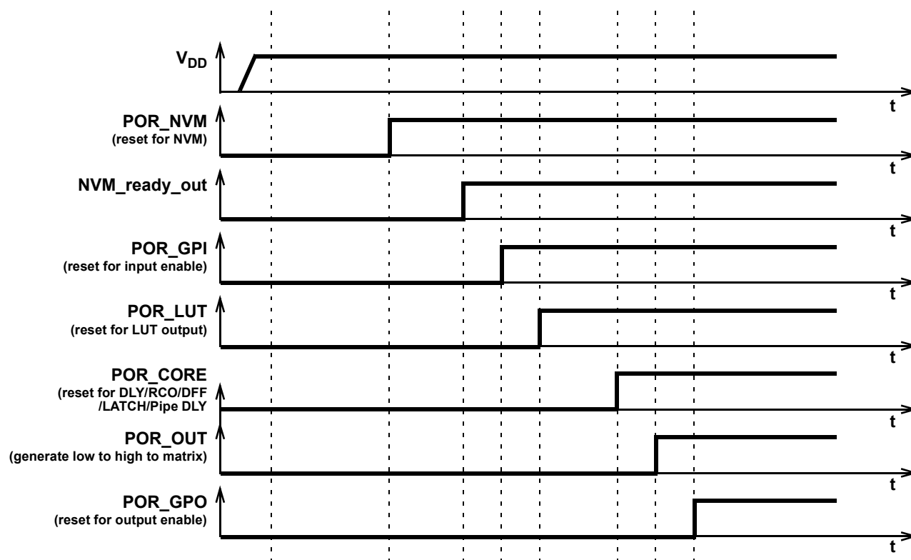
Figure 96: POR Sequence
