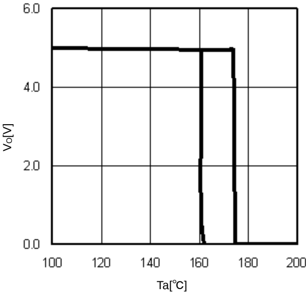
Fig.16 TSD ( I_o=0mA )
