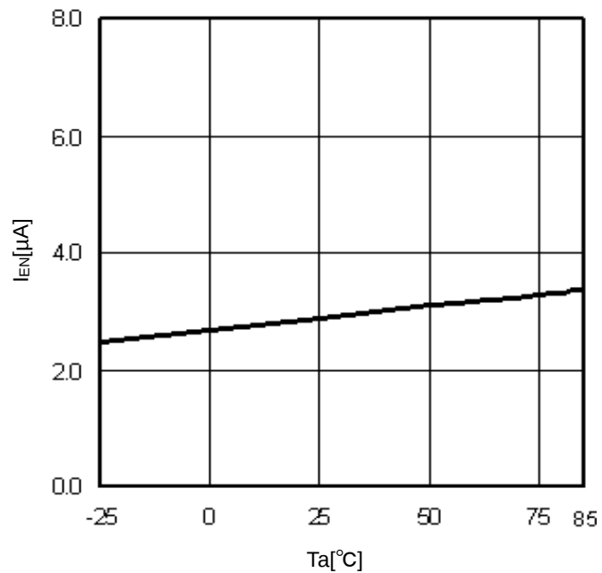
Fig.12 T_a - I_{EN}
