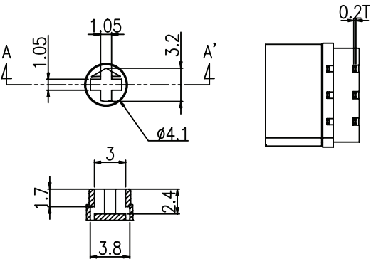
Section A-A' ACTUATOR
