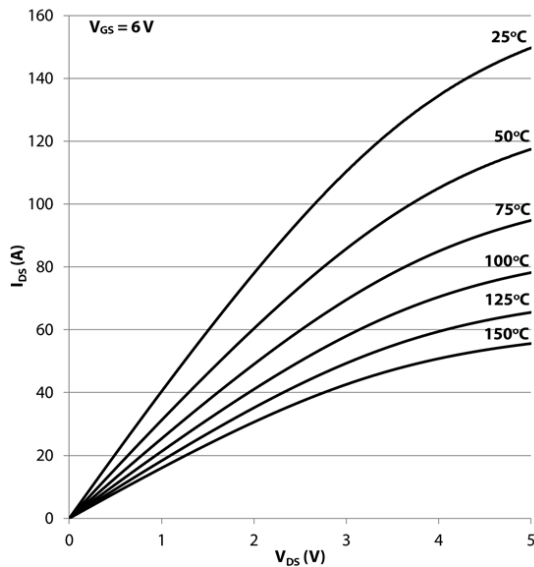
GS66516T I_{DS} vs. V_{DS} , T_J dependence
