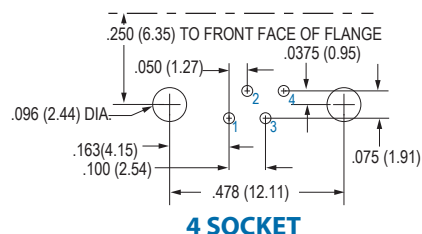
4 SOCKET
