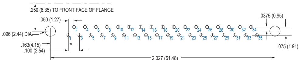
35 SOCKET
