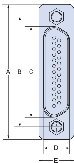
SOCKET
