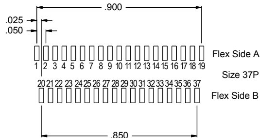
Size 37P
