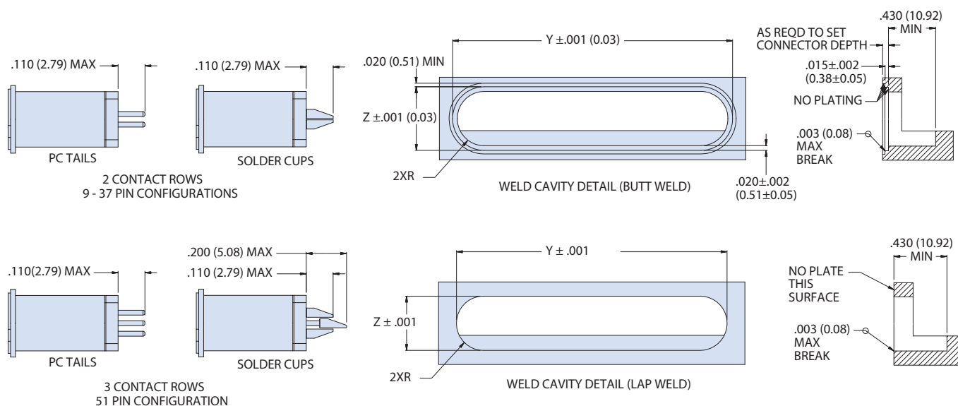
Cutout Dimensions
