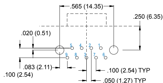
9 Socket
