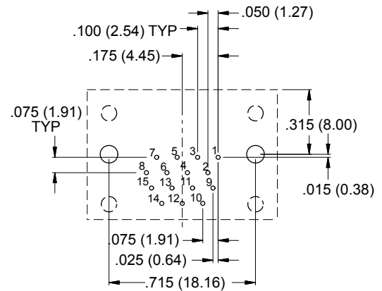
15 SOCKET
