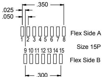
Size 15P
