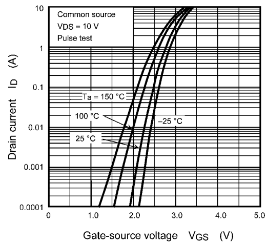
Fig. 8.2 I_D - V_{GS}
